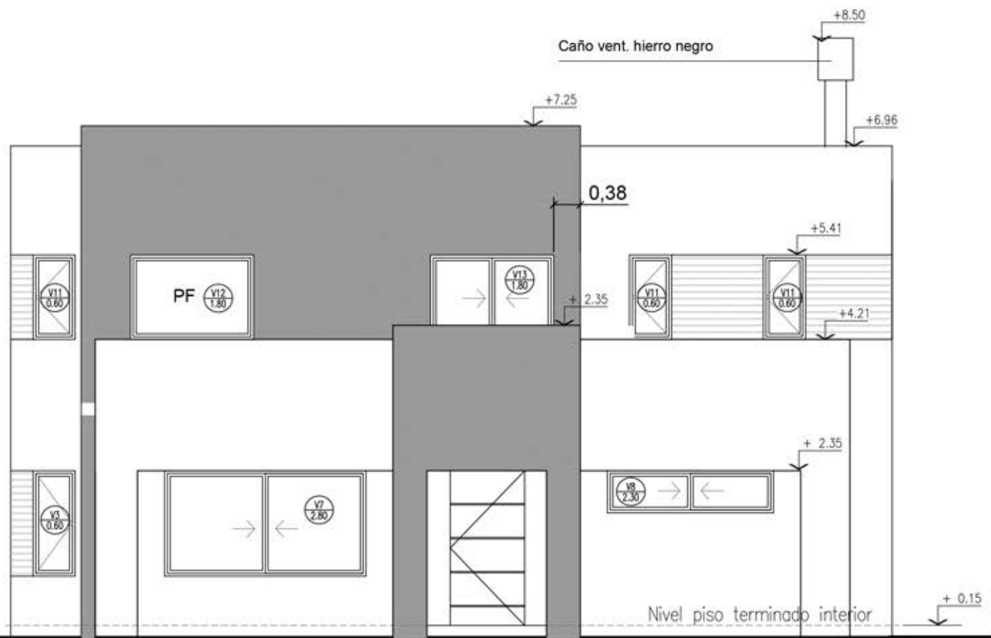
VISTA FRENTE
