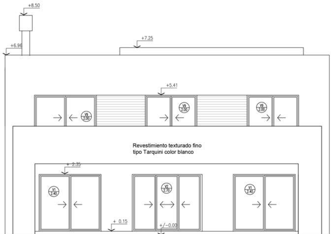
VISTA CONTRAFRENTE
